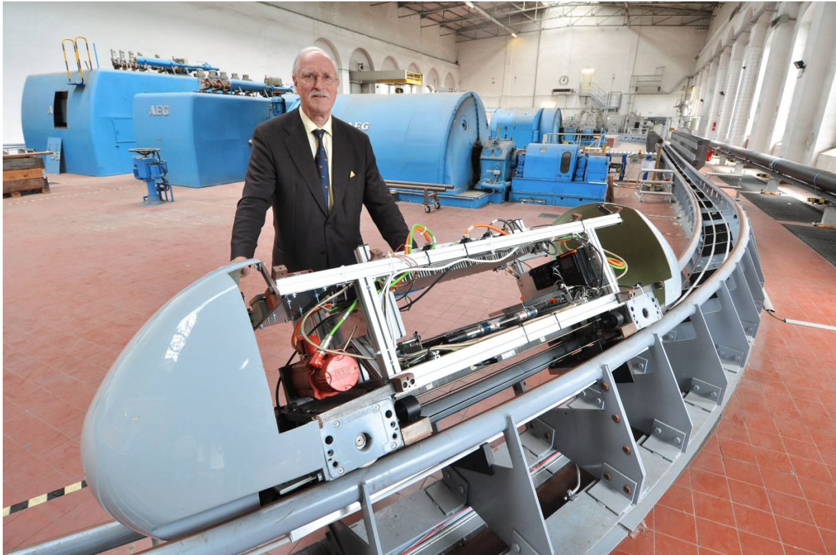
Bild: Prof. Dr.-Ing. habil. Dietrich Stein auf der CargoCap-Modellstrecke
